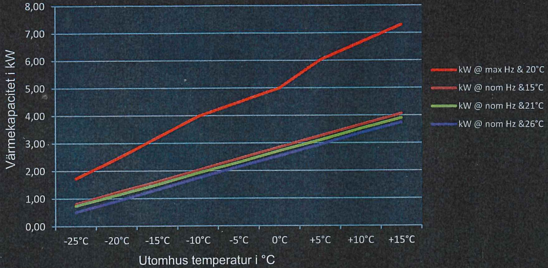
Värme kapacitet vs. utomhus temperatur MSZ-FH25VEHZ
