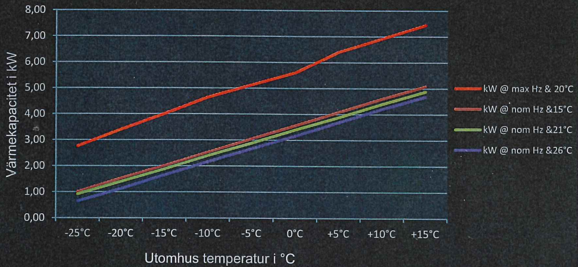
Värme kapacitet vs. utomhus temperatur MSZ-FH35VEHZ
